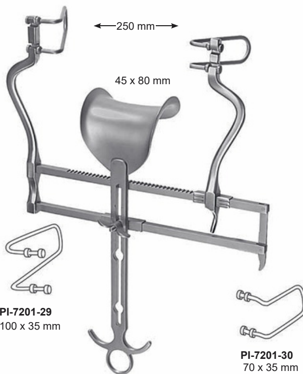
BALFOUR US-TYPE PI-7201-28
